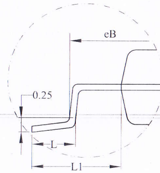
DETAIL: F
