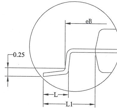
DETAIL: F
